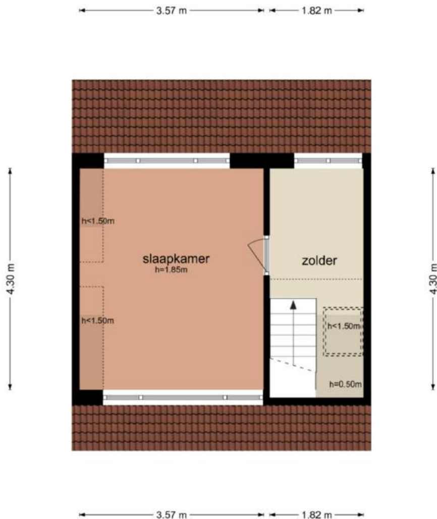
Maasstraat 7 - Nieuwegein Tweede Verdieping
